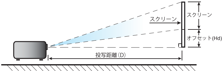
側面図
