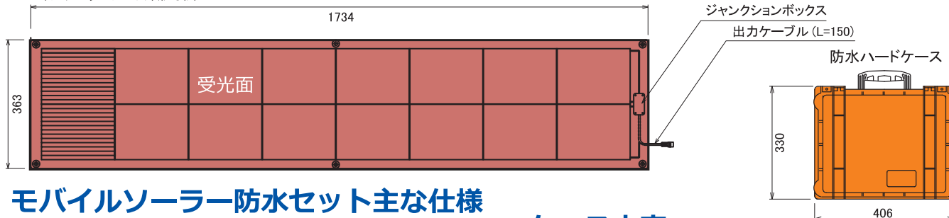
モバイルソーラーシート外形寸法
