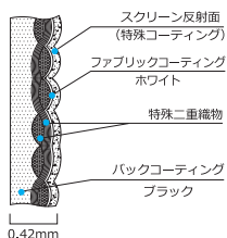
HF102 断面図
