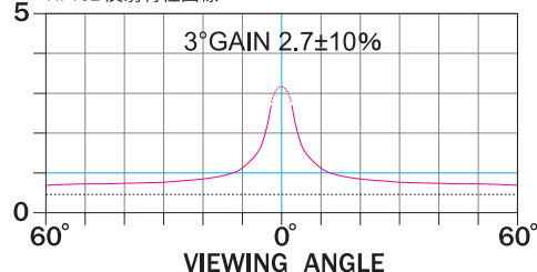
HF102 反射特性曲線
