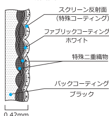
HF102 断面図
