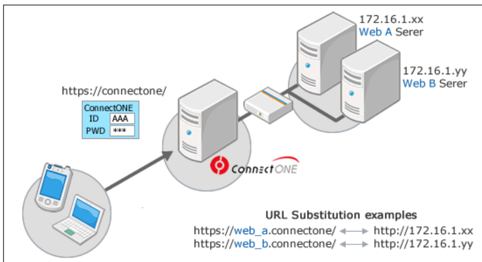
ConnectONE リバースプロキシ機能
