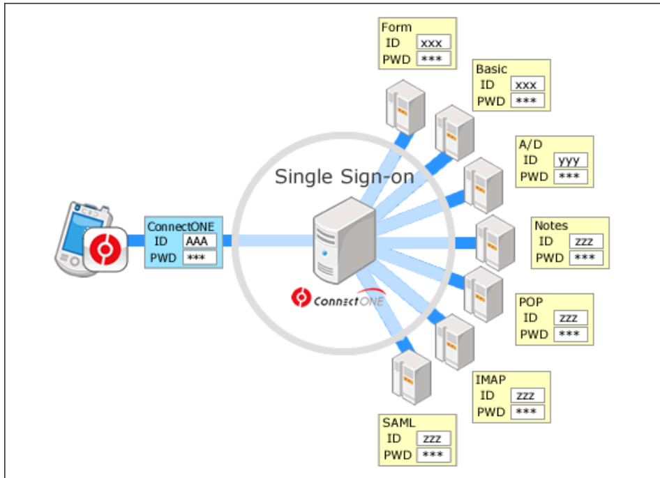
ConnectONE シングルサインオン機能
