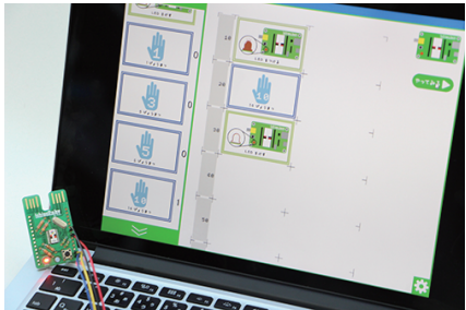
CutleryAppsの利用
