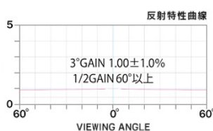
反射特性曲線
