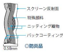
生地断面図
