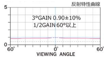
反射特性曲線
