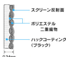
生地断面図
