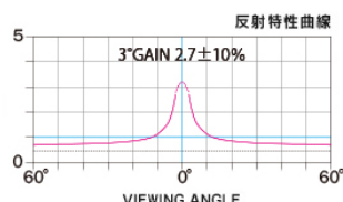
反射特性曲線
