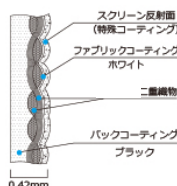
生地断面図
