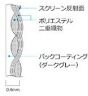
生地断面図
