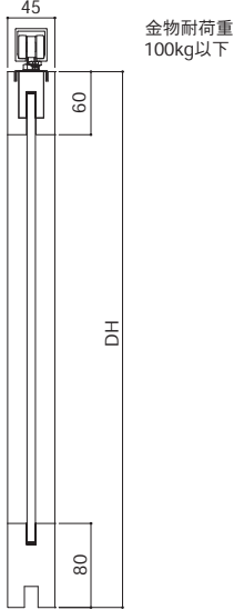
● 縦断面図
