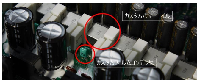
新開発フィルムコンデンサとカスタムパワーコイル
