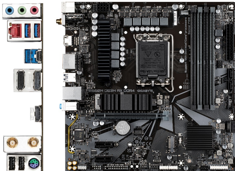
GIGABYTE B660M DS3H AX DDR4 Rev.1.0
