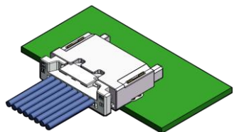
13103 シリーズ（1列品）
