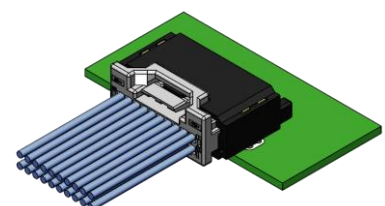
13065 シリーズ（2列品）
