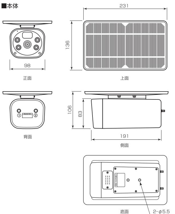
[寸法図] 単位:mm
