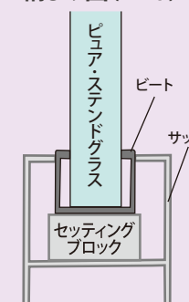
納まり図(ビート)
