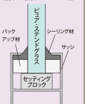
納まり図(シーリング材)
