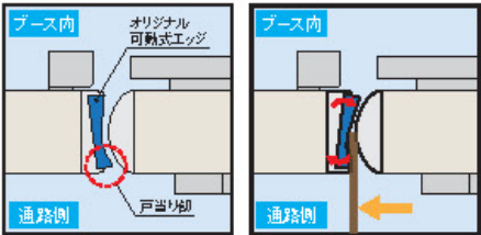
ドア戸先側 断面イメージ
